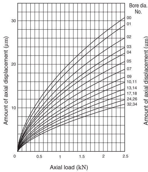
(4) 7000 (contact angle 30°)
